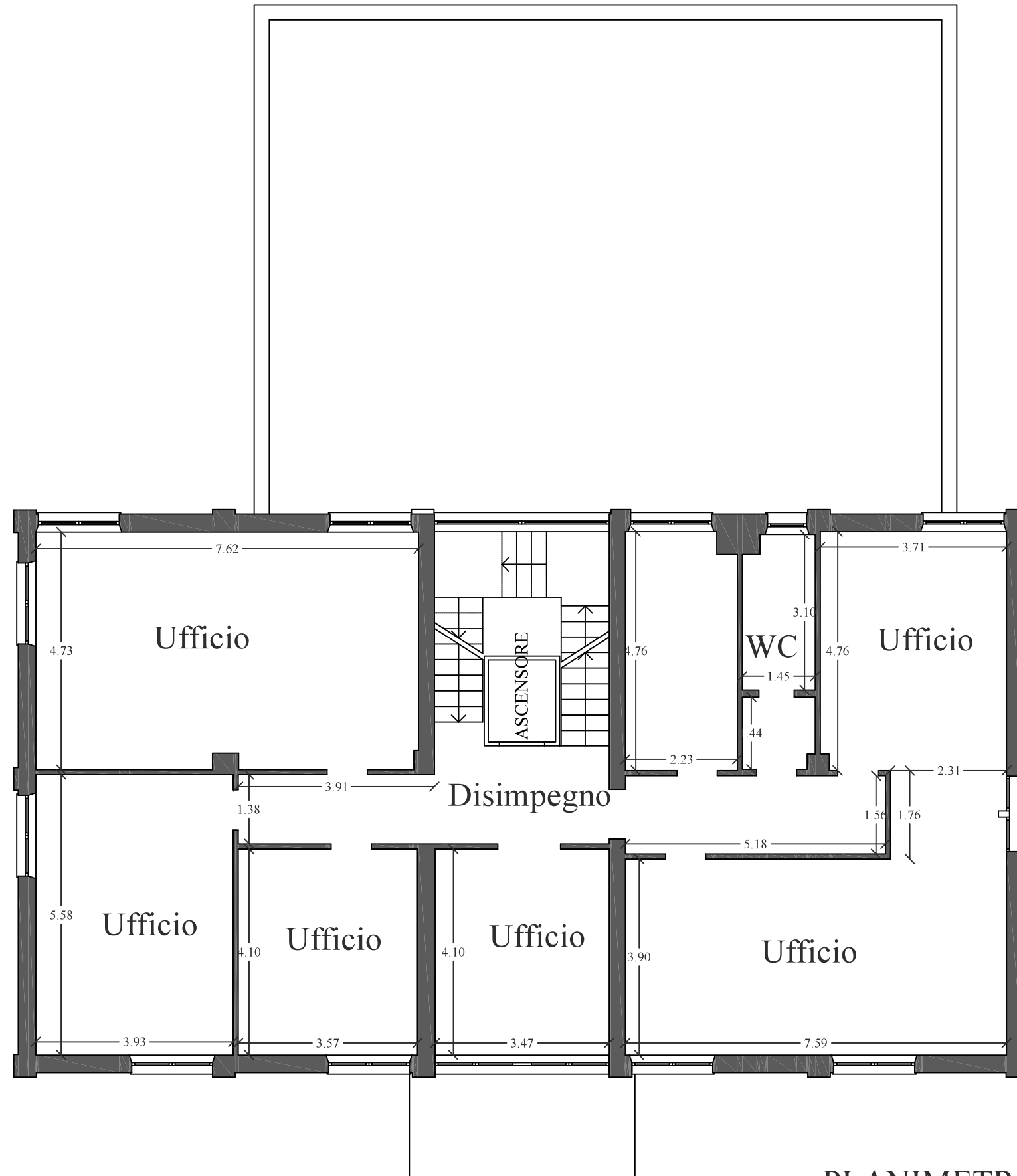
PLANIMETRIA PIANO PRIMO Scala 1:100
